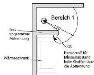
4) Draufsicht (mit fest angebrachtem Wasserauslass sowie fest angebrachter Abtrennung und Radius für Mindestabstand beim Greifen um die Abtrennung herum)
