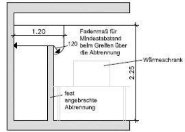
2) Seitenansicht (mit fest angebrachter Abtrennung sowie Radius für den Mindestabstand beim Greifen über die Abtrennung)
